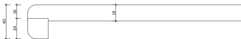
1 01 Fensterbank Typ 142 Blende 40 mm
