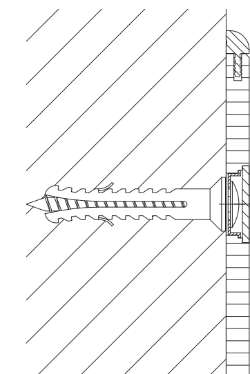
4. ... LEICHT ANDRÜCKEN
