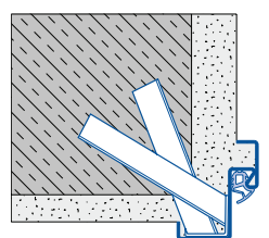
Pose avec pattes d'ancrage murales
