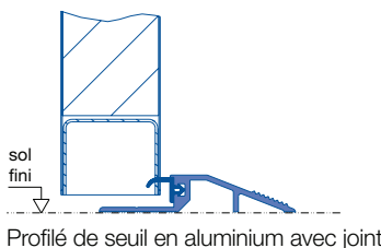
Profilé de seuil en aluminium avec joint
