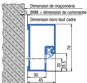
Huisserie tubulaire pour pose dans la baie (profilé 21101)
