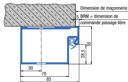
Huisserie tubulaire pour montage en applique (profilé 006)
