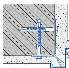
Pose avec pattes d'ancrage à cheviller
