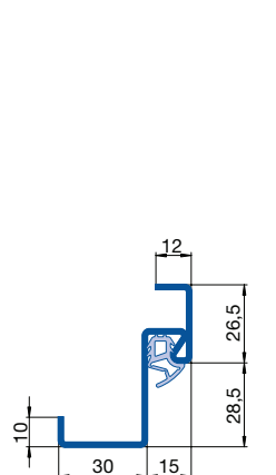
Huisserie d'angle de série
