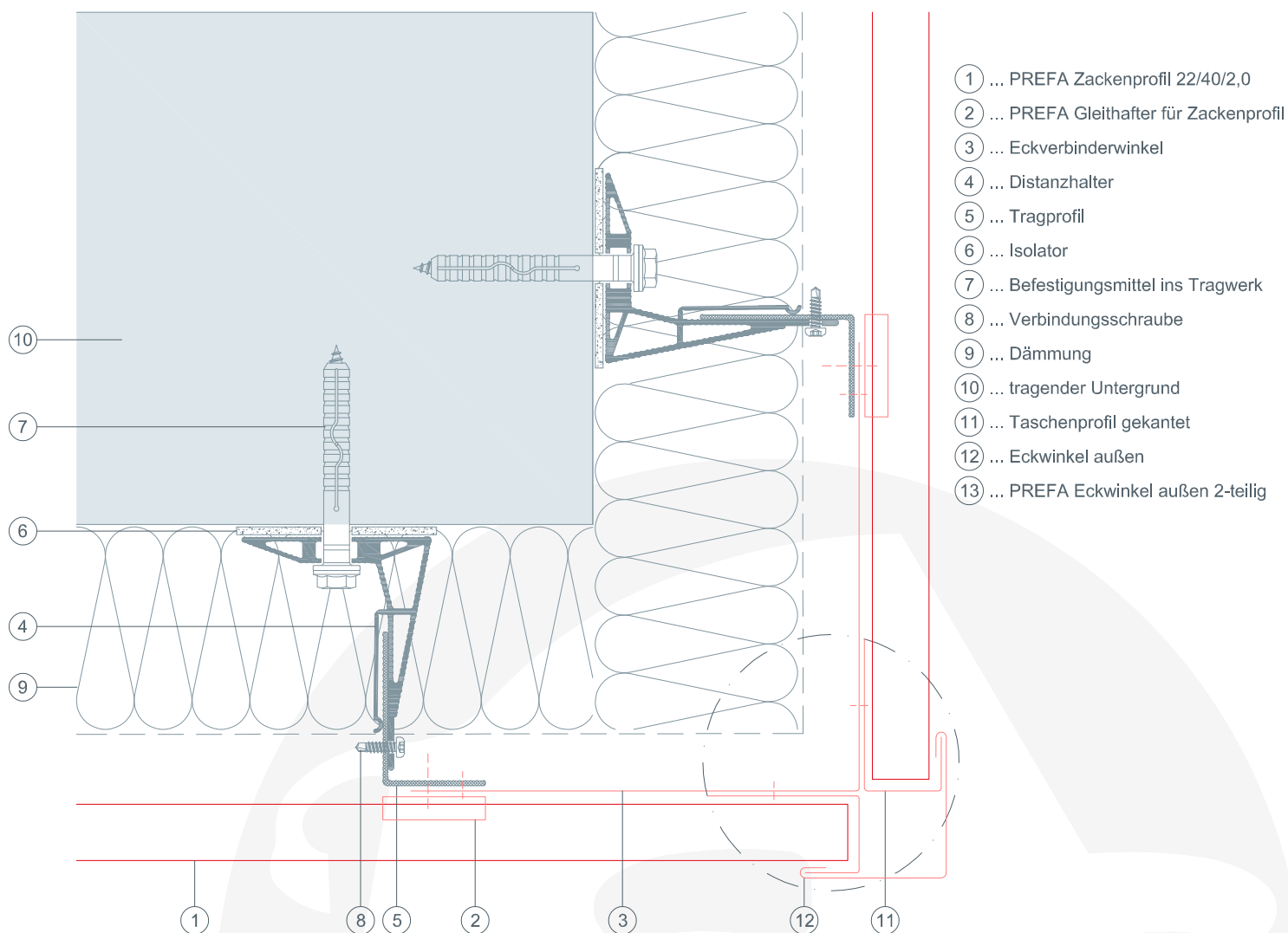
Anschlussvariante
