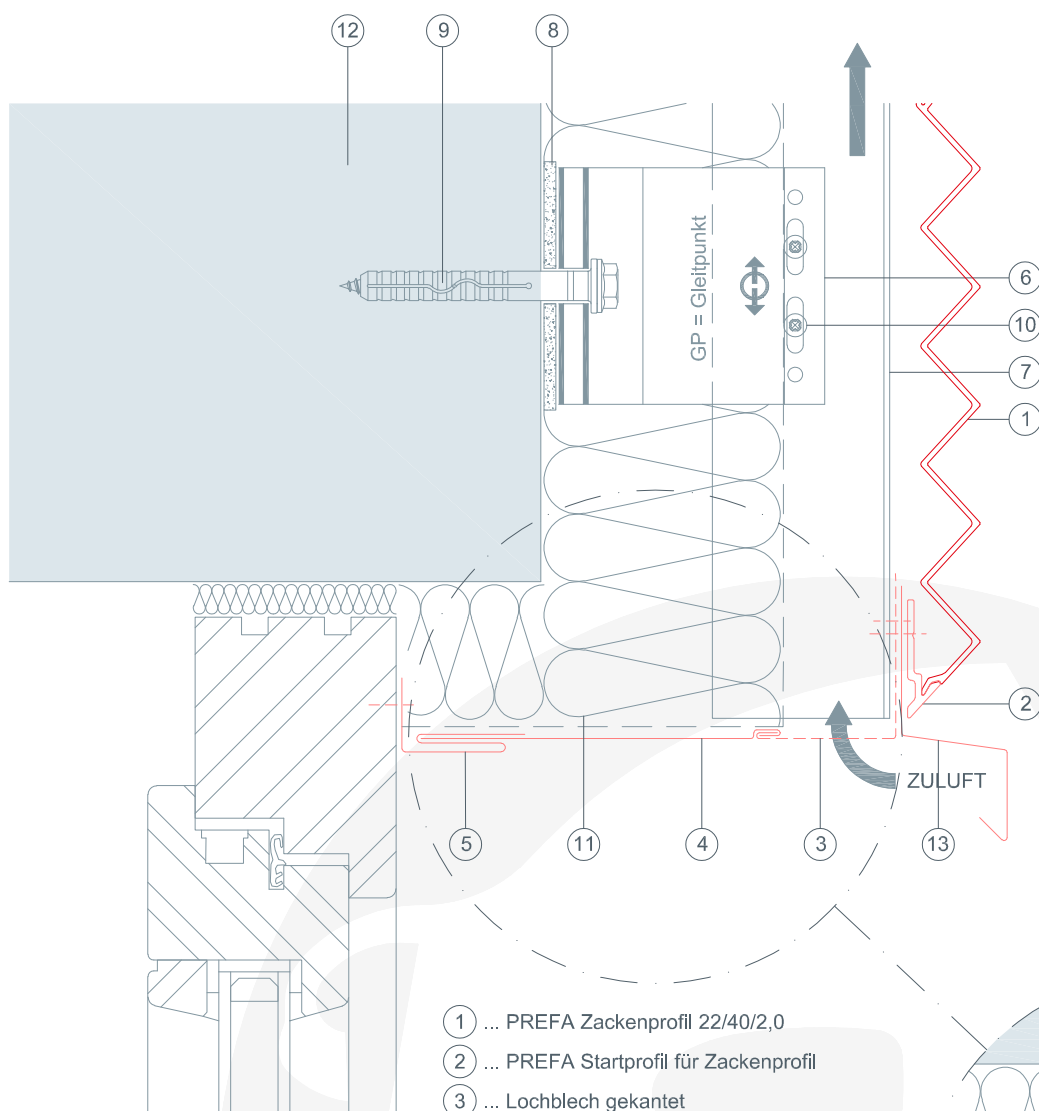
Anschlussvariante
