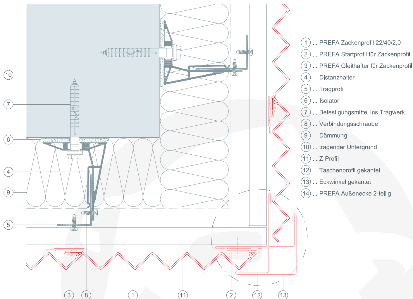
Anschlussvariante
