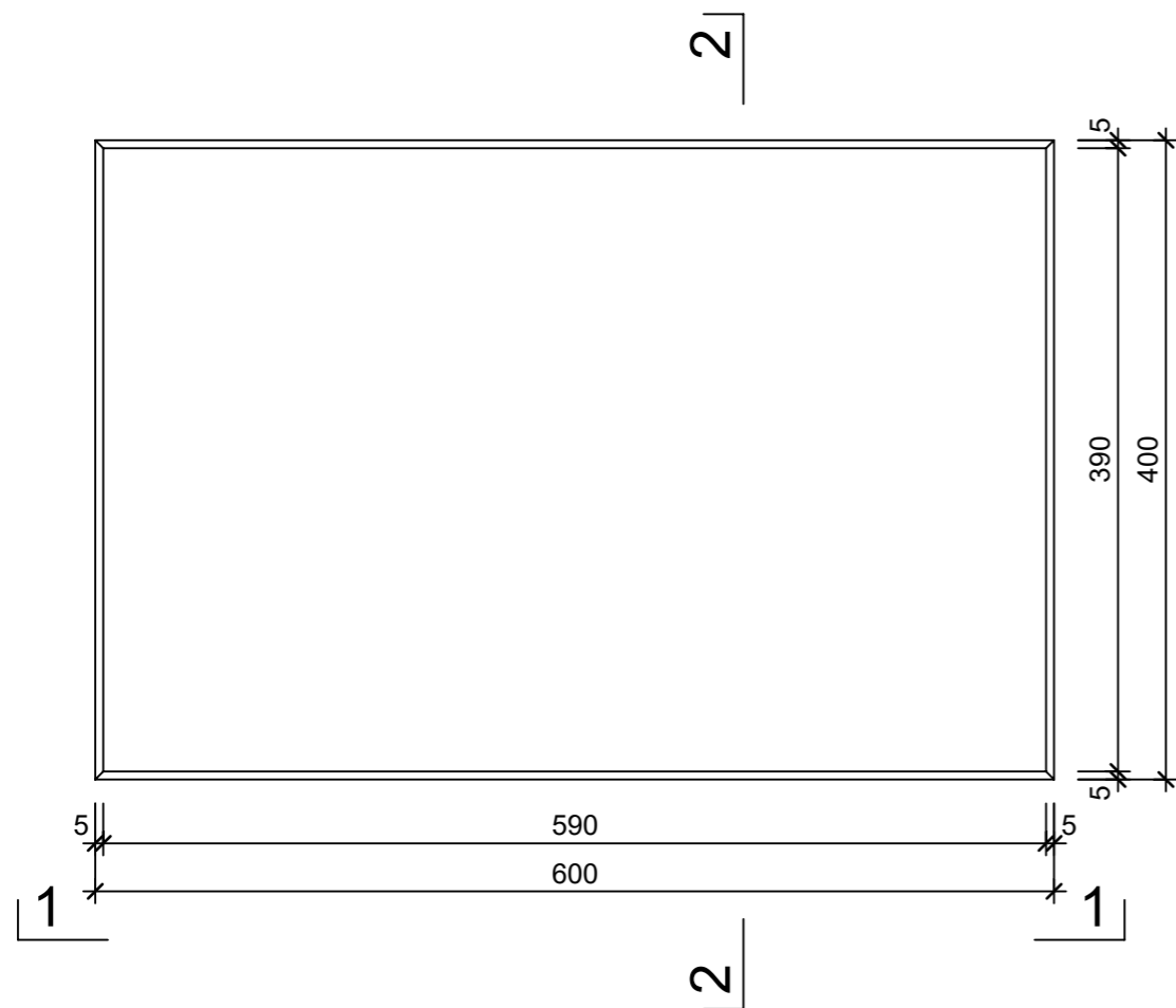
Grundriss, 1:5
