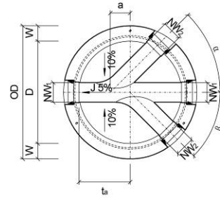
Bild 6: Grundriss CRENO Normschachtboden Typ 2
