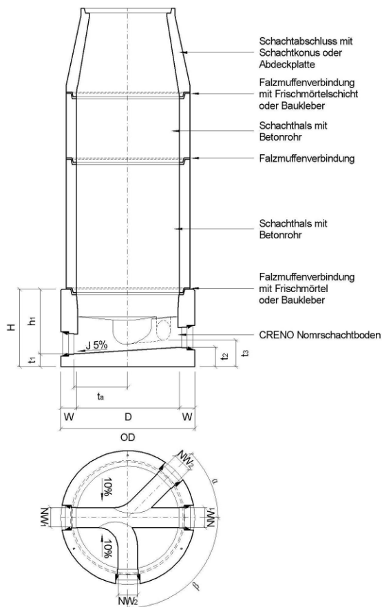
Bild 3: Beispiel eines Längsschnittes eines CRENO Normschachtes
