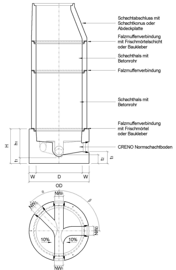
Bild 4: Beispiel eines Querschnittes eines CRENO Normschachtes
