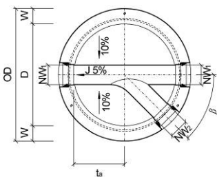
Bild 9: Grundriss CRENO Normschachtboden Typ 5
