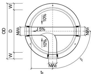
Bild 11: Grundriss CRENO Normschachtboden Typ 7
