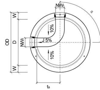
Bild 14: Grundriss CRENO Normschachtboden Typ 10
