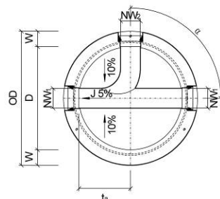
Bild 12: Grundriss CRENO Normschachtboden Typ 8
