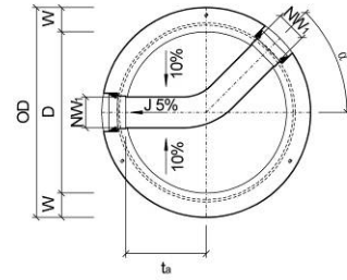
Bild 16: Grundriss CRENO Normschachtboden Typ 12
