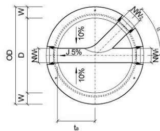
Bild 10: Grundriss CRENO Normschachtboden Typ 6
