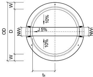
Bild 5: Grundriss CRENO Normschachtboden Typ 1
