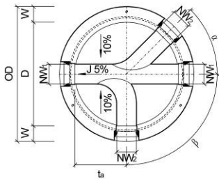
Bild 7: Grundriss CRENO Normschachtboden Typ 3
