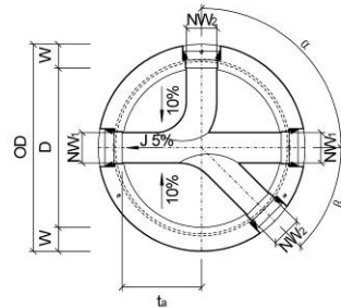
Bild 8: Grundriss CRENO Normschachtboden Typ 4
