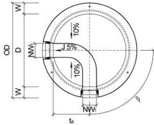
Bild 13: Grundriss CRENO Normschachtboden Typ 9
