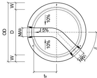
Bild 15: Grundriss CRENO Normschachtboden Typ 11
