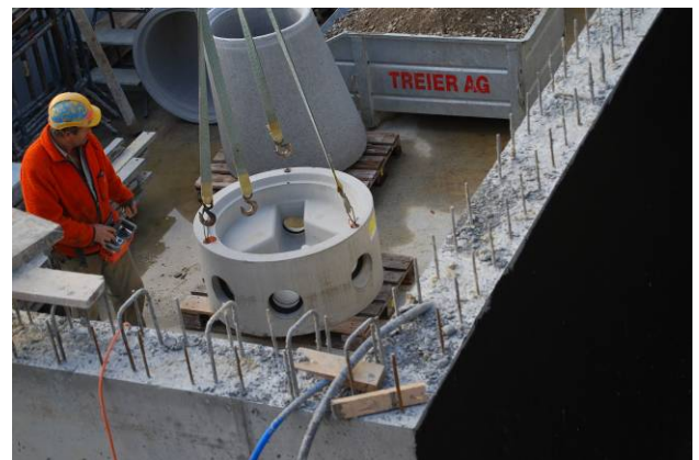
Bild 21: Lagerung auf der Baustelle
