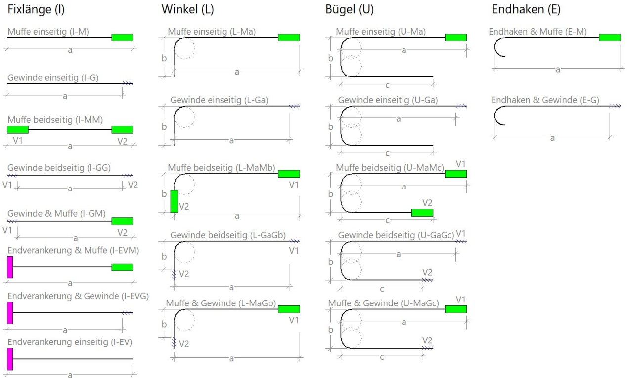
Ma: Muffe bei Seitenlänge a / Gb: Gewinde bei Seitenlänge b
