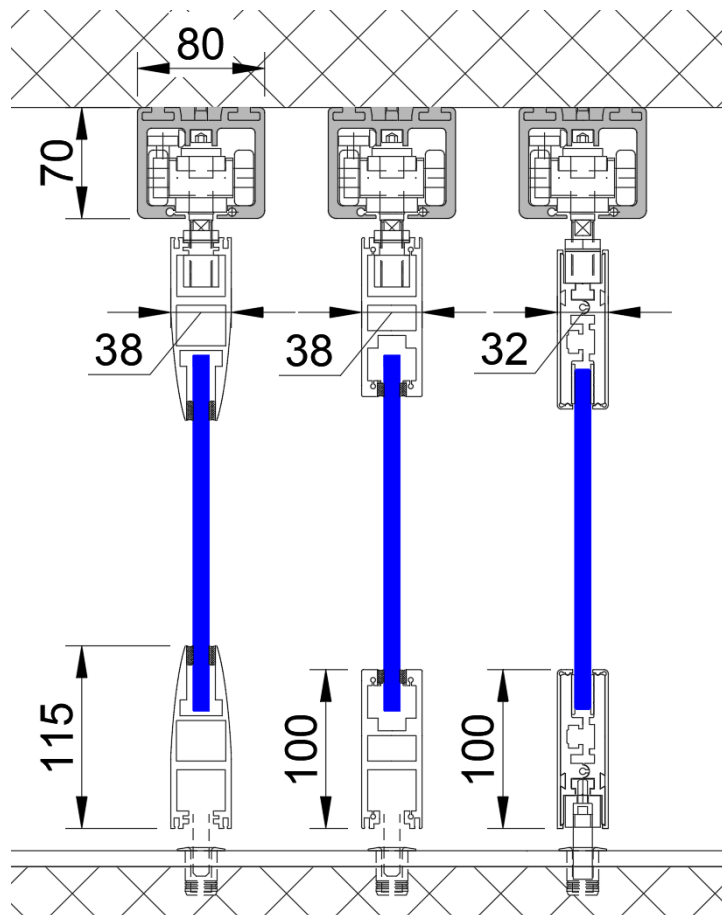
Typ D
