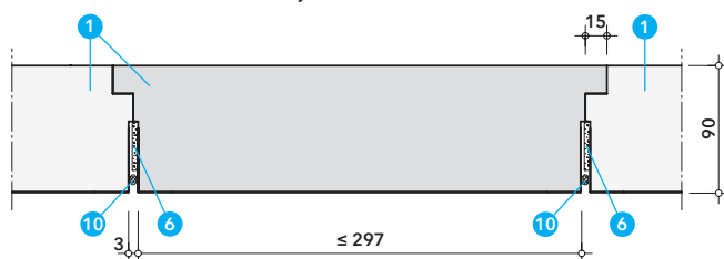
joint de l'élément
