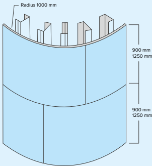
Ausführung mit voller Plattengrösse für r ≥ 1.0 m
