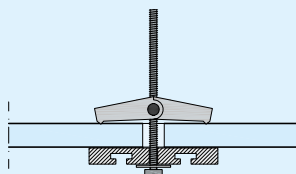
Federklappdübel z.B. Vorhangschiene
