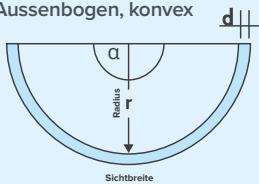
Aussenbogen, konvex
