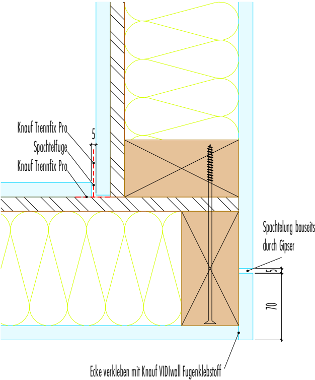
Eckausführung Variante 2
