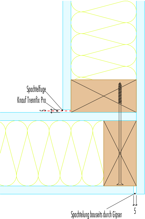
Eckausführung Variante 3
