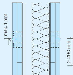
1. Untere Lage stumpf gestossen 2. Äussere Lage mit Klebefuge
