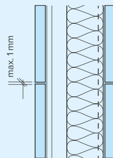
Horizontale Klebefuge
