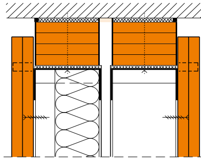
fermacell™ Montagewand als Doppelständerwand, zweilagig beplankt, gleitender Deckenanschluss
