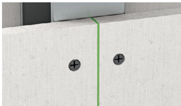
fermacell™ Klebefuge – Fugenbreite: \leq 1 \text{ mm}
