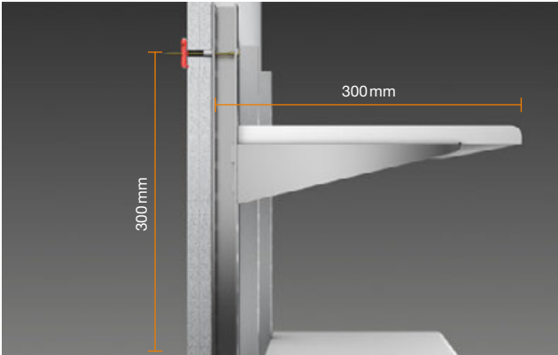
Einzelaufhängung jeweils mittig zwischen Unterkonstruktion angeordnet
