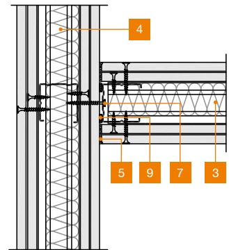
1 S 31 fermacell™ Montagewand
