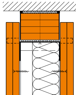
fermacell™ Montagewand, zweilagig beplankt, gleitender Deckenanschluss
