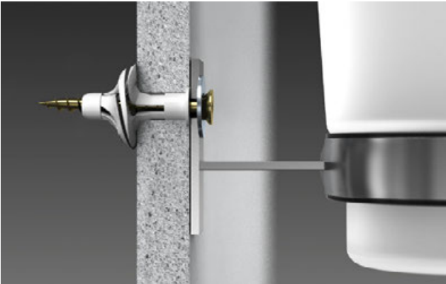
Lastenbefestigung mit Dübel an Trockenbauwand
