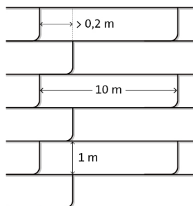
Vermeidung von Kreuzstößen
