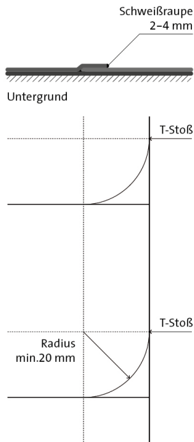
Die sichtbaren Ecken der Abdichtungsbahnen sind abzurunden
