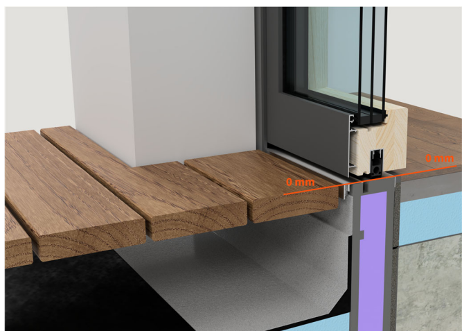
windura classic seuil zéro
