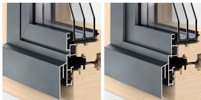
Vantail à arêtes vives, affleuré ou décalé du cadre
