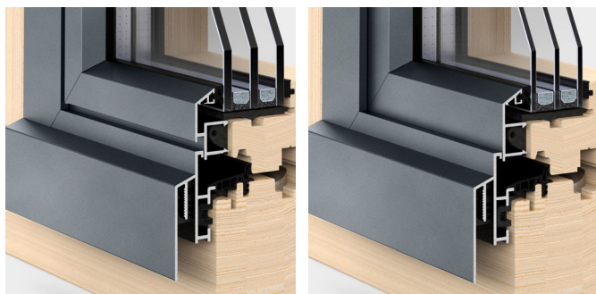
Vantail à arêtes en biais, affleuré ou décalé du cadre
