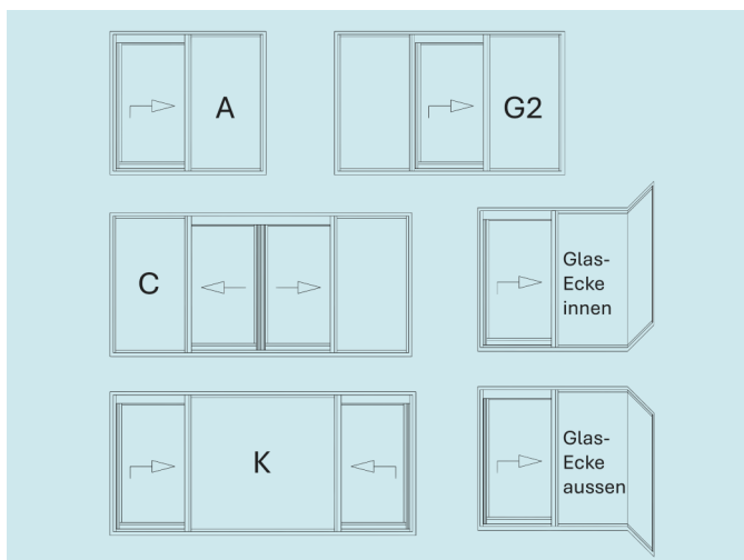
Öffnungsschemen
