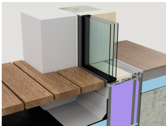
Festverglasung, Panoramaverglasung
