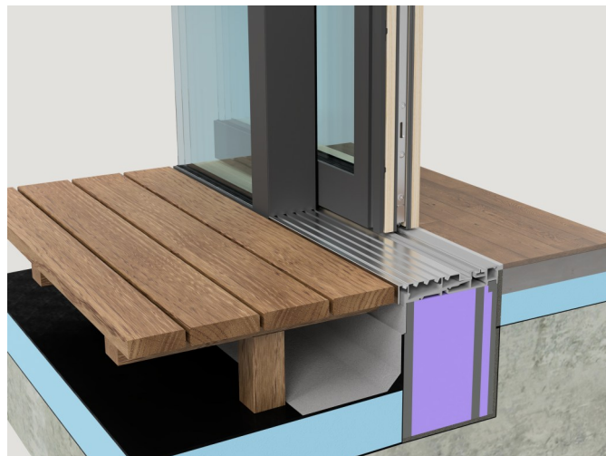
duraslide top
