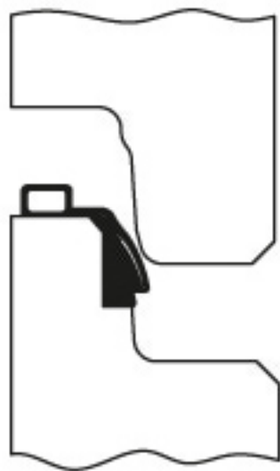
Selbst- schmierende Keilgleit- dichtung
