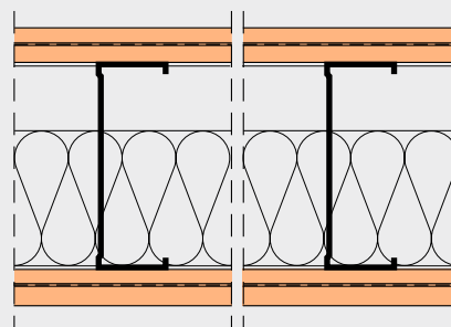
fermacell Brandwand tragend 4 S 33
