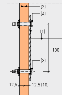
Beispiel: Fernseh-/Monitorkonsole
