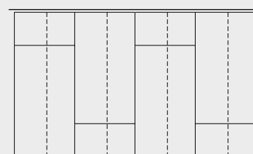
Anordnung der Plattenstöße bei einlagiger fermacell Beplankung
