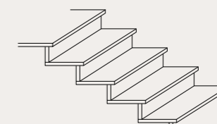
c) Scala classica appoggiata con frontale
