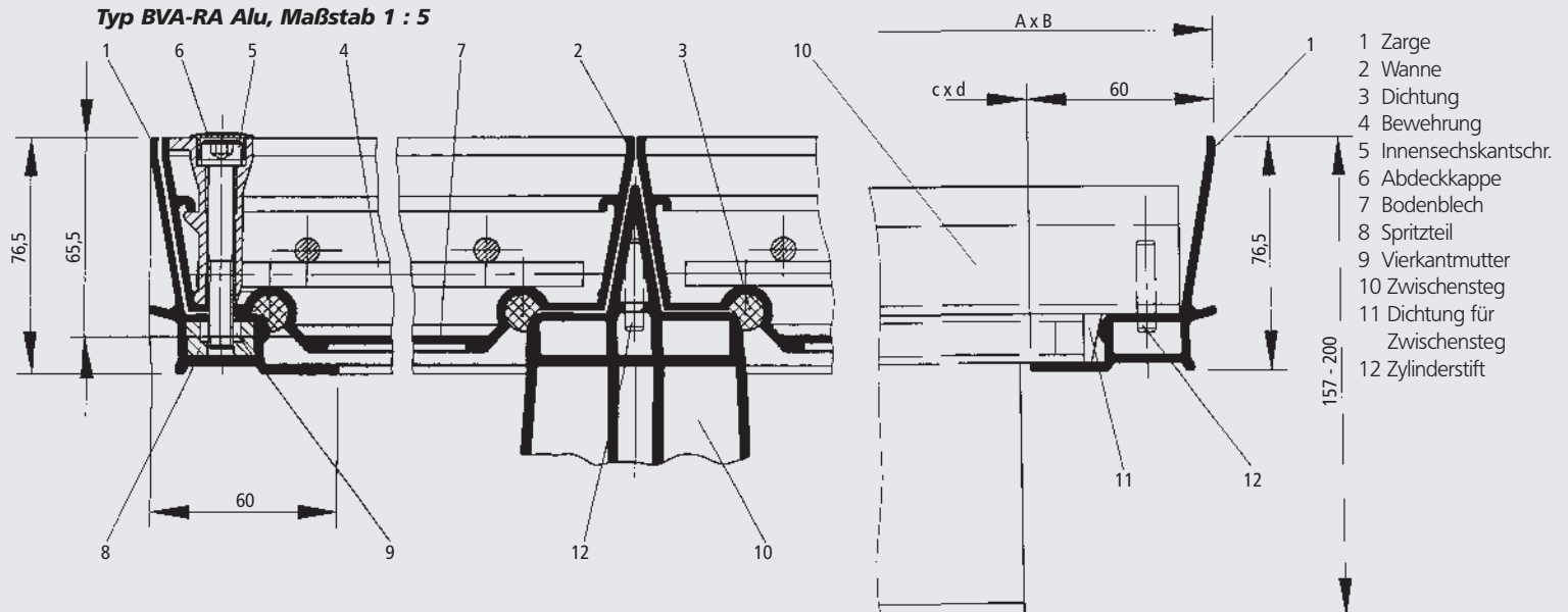
Detail Abzweigung
