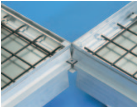
Detail Abzweigung
