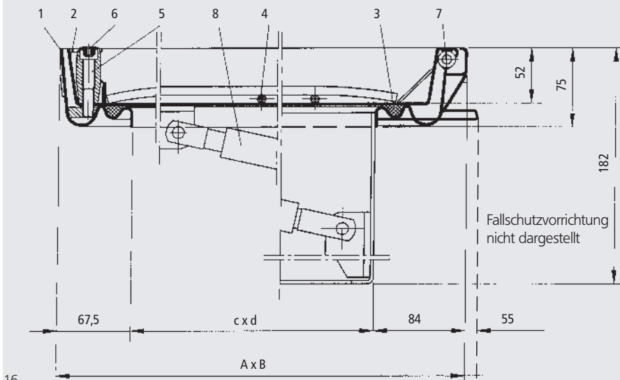
Typ BV-GD Stahl/BVE-GD Edelstahl, Maßstab 1 : 5
