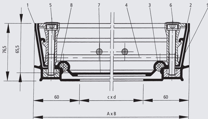
Type BVA aluminium, Échelle 1 : 2,5
