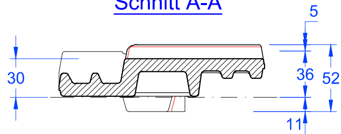
Schnitt A-A
