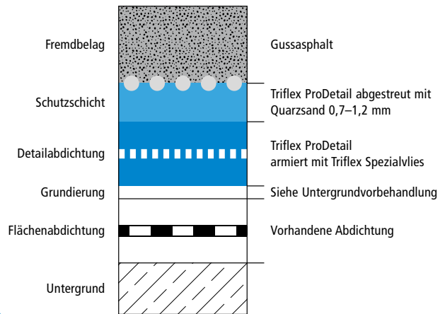
Systemaufbau – Detail D
