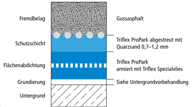
Systemaufbau – Detail A
