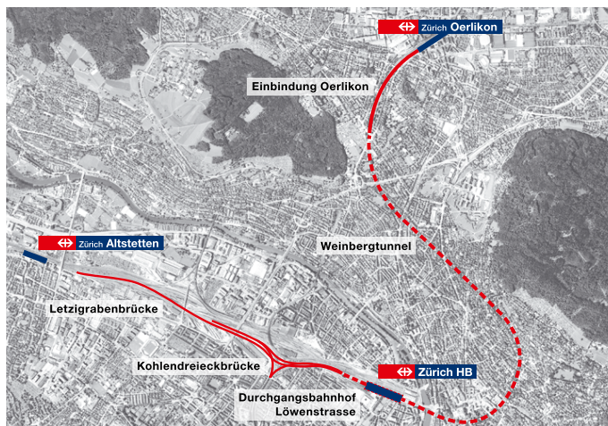
Übersicht Gesamtprojekt Durchmesserlinie
