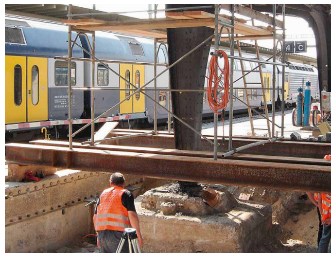
Bauarbeiten im laufendem Bahnbetrieb
