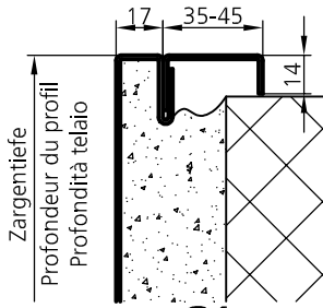
Variante: G1 (ST7.UD.G1)
