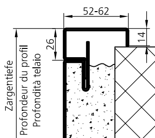
Variante: E1 (ST7.UDS.E1)
