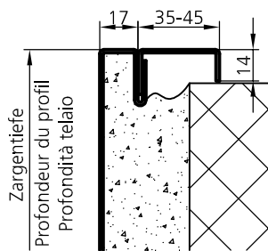
Variante: G1 (ST7.UDS.G1)
