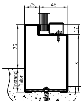
Sockel mit Bodeneinstand Socle avec talon
