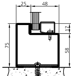
Sockel ohne Bodeneinstand Socle sans talon
