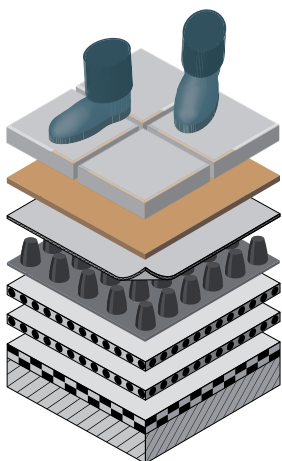
Aufbau Nophadrain Terrassensystem mit ND 220 Drainagesystem
