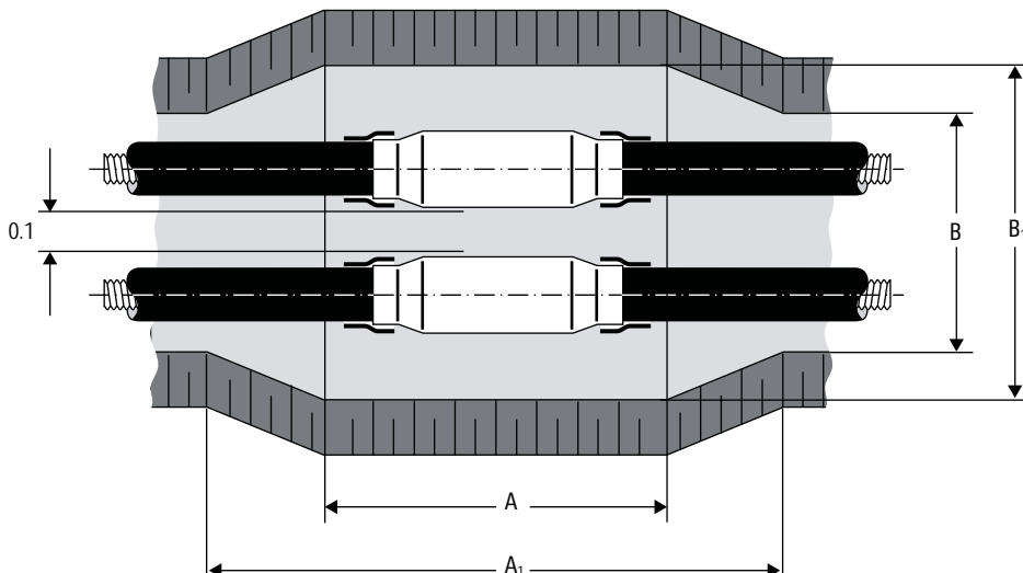
Fig.2: spazio di lavoro per raccordo passante (vista dall'alto)
