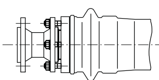
Tipo DE Versione speciale per installazioni sanitarie Dimensioni del raccordo a flangia secondo PN 16
