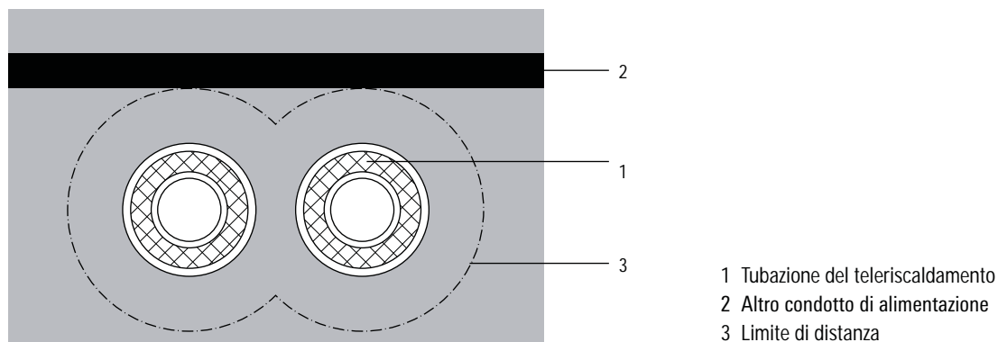
Fig. 1: tubazioni incrociate
