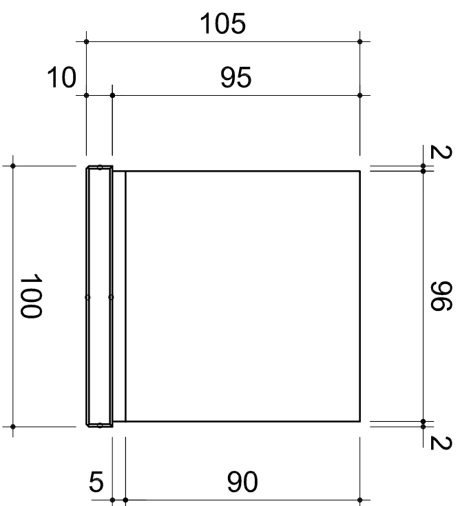
Grundriss 1:20
