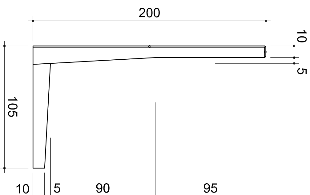
Querschnitt 1:20
