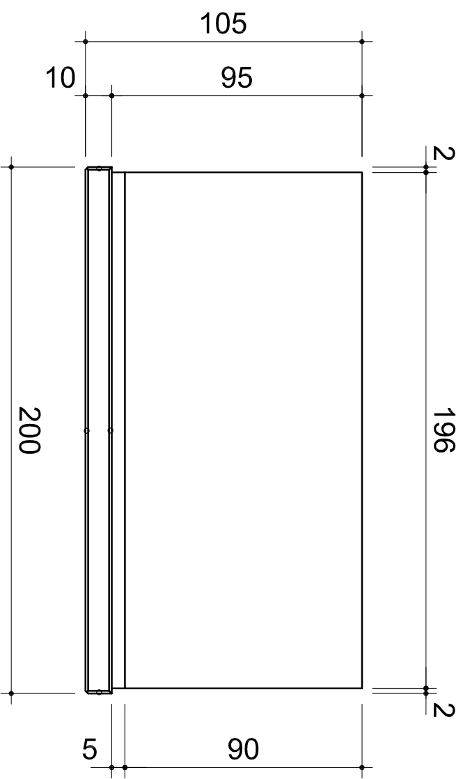
Grundriss 1:20
