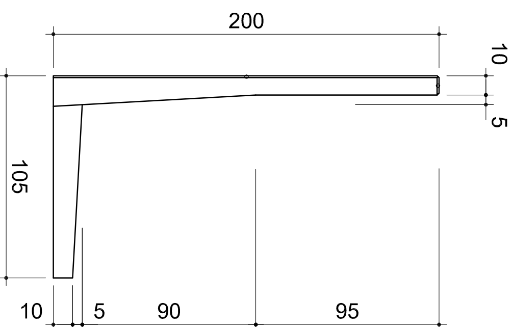
Querschnitt 1:20
