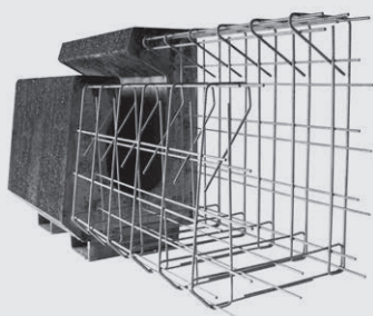
Caniveaux de drainage
