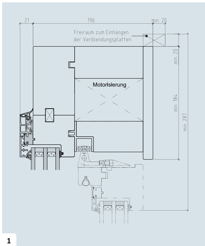
1 Festteil, Schnitt oben, Typ GL
