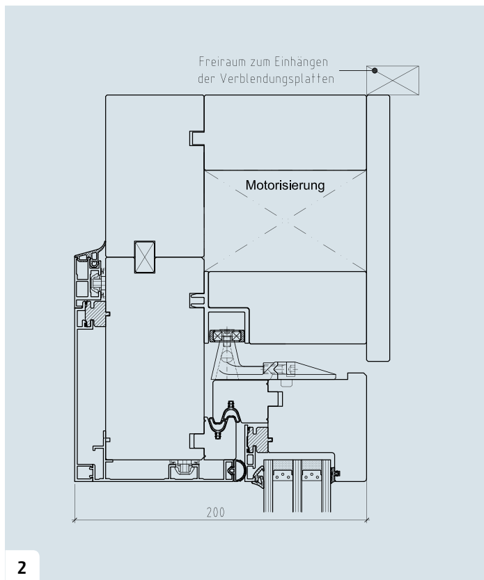
2 Durchgang, Schnitt oben
