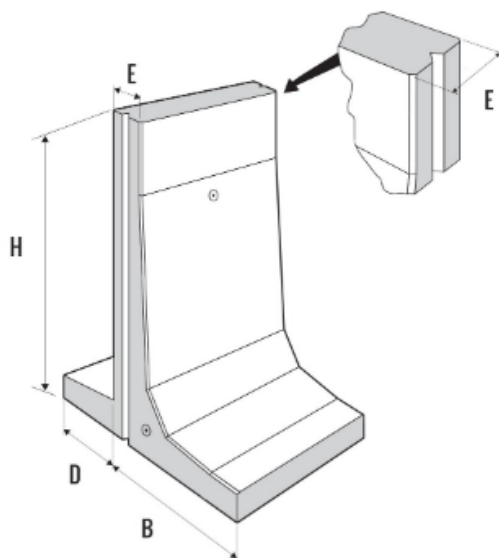
PROFIL EN T
