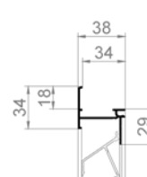
G 30Z Grille murale à encaster avec aile de recouvrement
