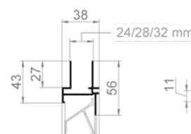
F 30Z Grille de fenêtre
