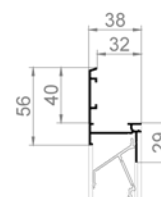
G 30Z Large Grille murale à encaster avec aile de recouvrement extra large
