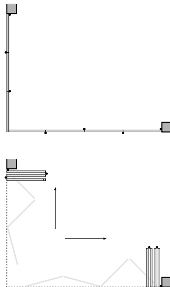
Pfostenlose Eckerlage
