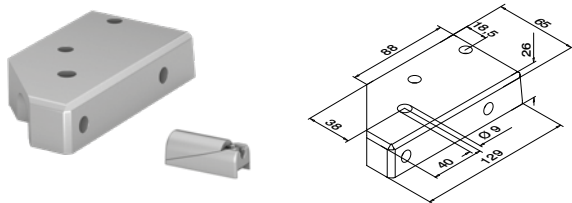
Außenecke Links Inklusive Nivellierblock
